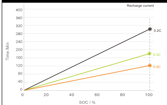
Temps de charge typiques
